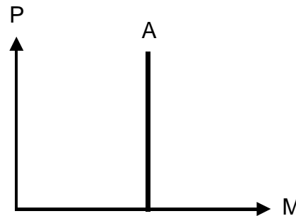
25 Vollkommen unelastisches A (e=0)
